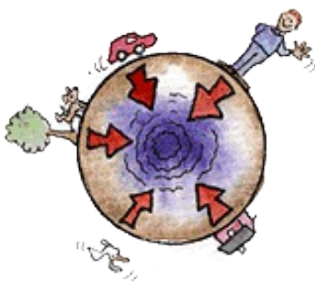
Dragningskraft/tyngdkraft
